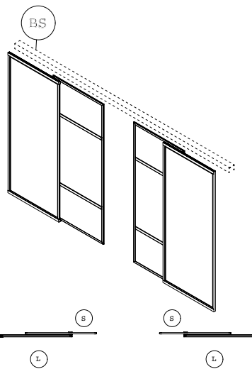
Configurazione angolo + anta scorrevole / Corner + sliding door configuration
