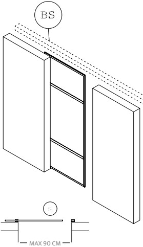
Configurazione anta scorrevole singola / Single sliding door configuration
