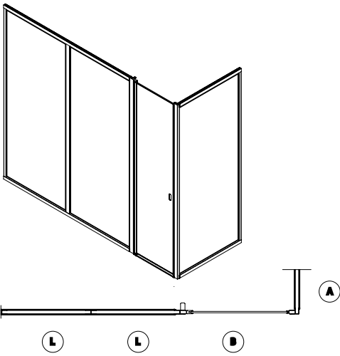
Configurazione per pannelli in linea + porta a battente + angolo / Fixed panel + swing door + corner configuration
