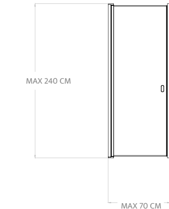
PORTA CON MANIGLIA / Door with handle
