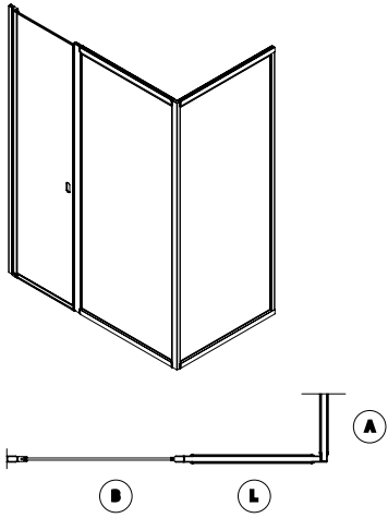
Configurazione porta a battente + pannello + angolo / Swing door + fixed panel + corner configuration
