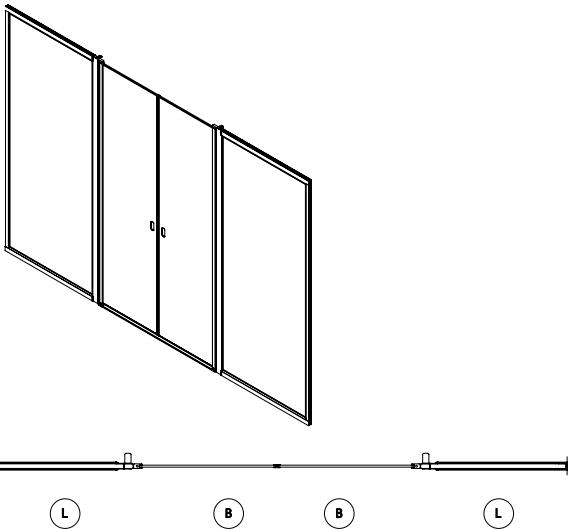
Configurazione pannelli in linea con doppia porta a battente centrale / Fixed panels with central double swing door
