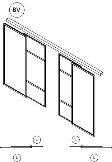
Configurazione anta scorrevole singola / Single sliding door configuration
