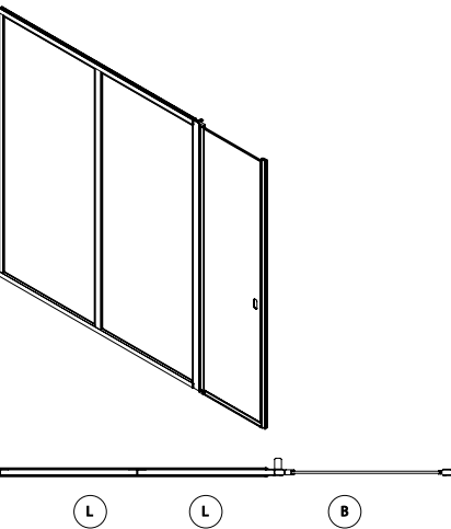
Configurazione pannelli in linea + porta a battente / In-line fixed panels + swing door configuration
