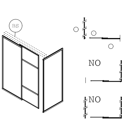
Configurazione angolo + anta scorrevole / Corner + sliding door configuration
