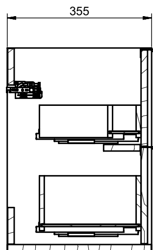
B-B ( 1 : 7 )
